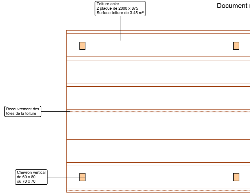
Plan de la toiture et de l'emplacement des chevrons verticaux
