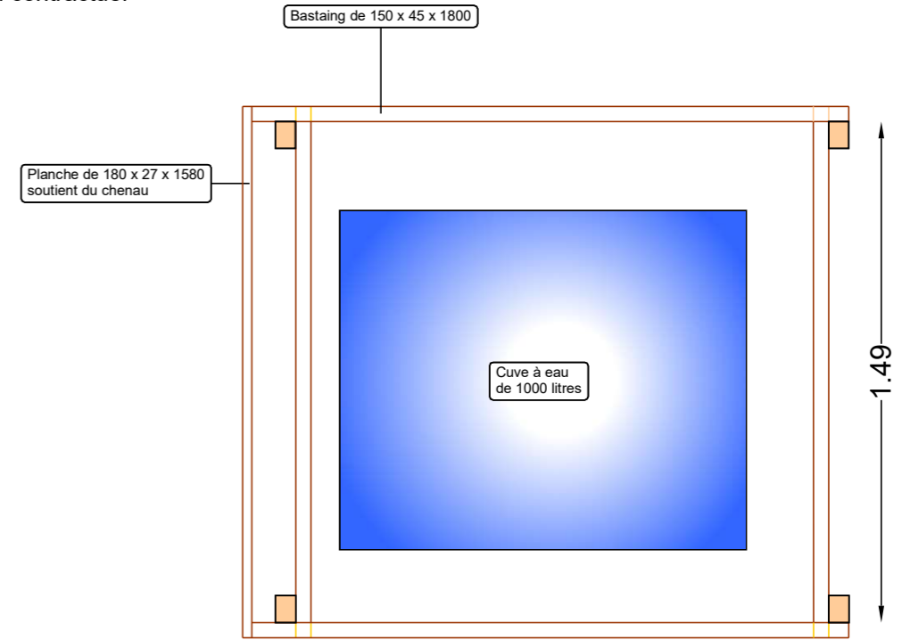
Plan de l'emplacement du coffre et cuve
