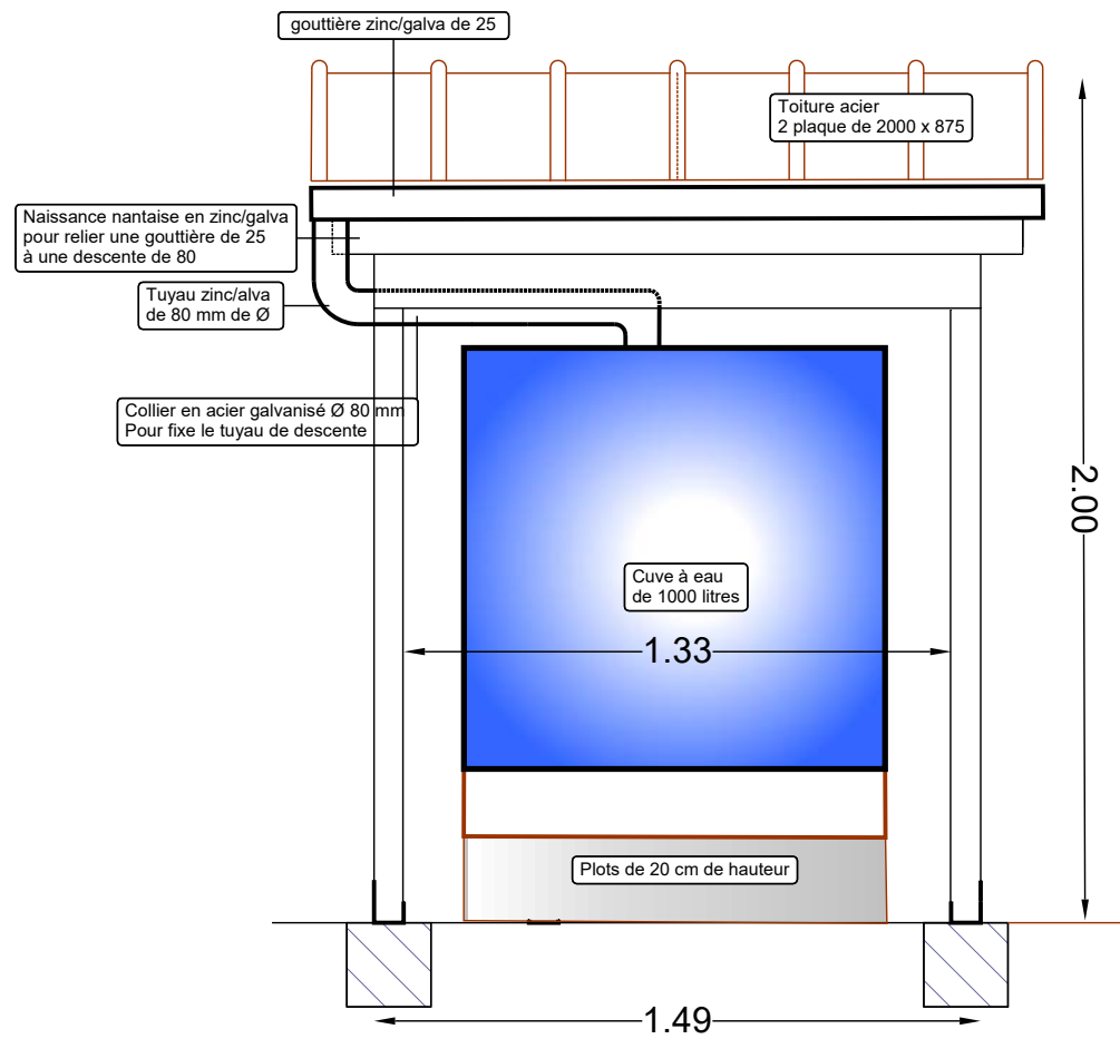
Facade arrière Zinquerie
