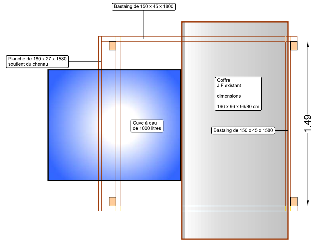
Plan de l'emplacement du coffre et cuve ( version coffre JF)
